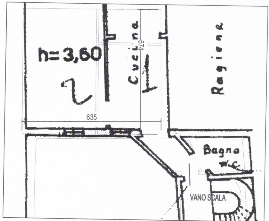
APPARTAMENTO - SUB. 5 SOVRAPPOSIZIONE PLANIMETRIA CATASTALE E RILIEVO DELLO STATO DI FATTO scala 1:100
